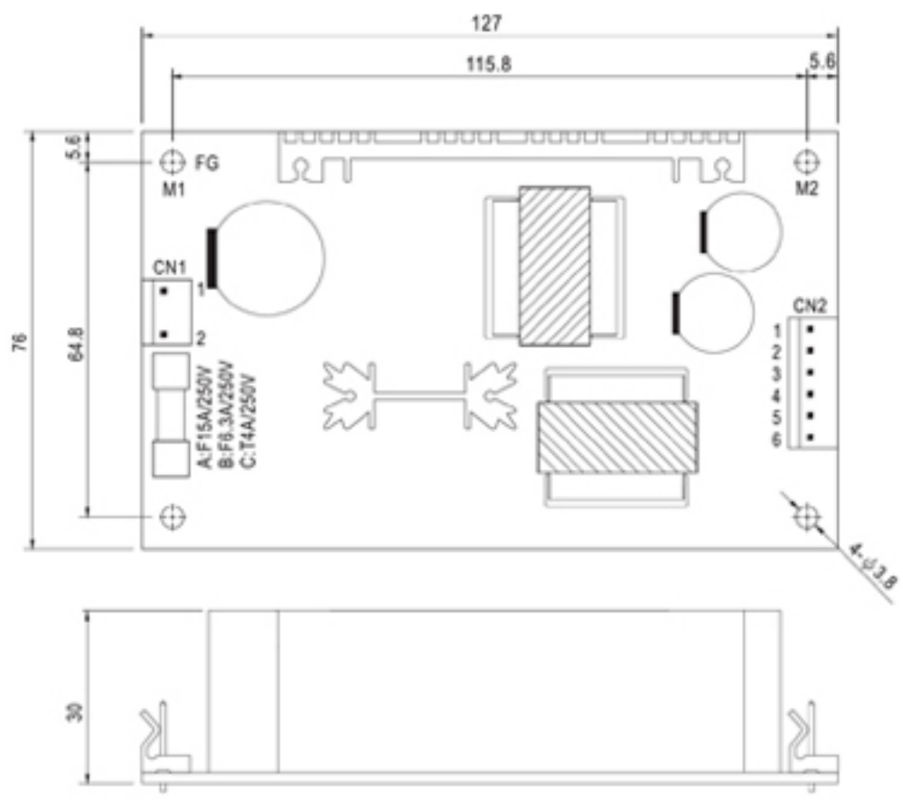
DC直流输入连接器(CN1): Molex 5277-02或等同型号
